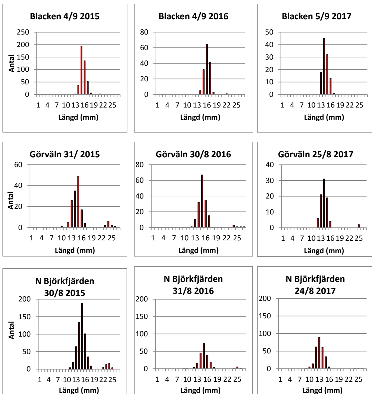
Figur 15. Längdfördelning hos M. relicta s.l. i håvprov insamlade i de tre Mälarfjärdarna Blacken, Görväl och Norra Björkfjärden i slutet av augusti/början av september 2015-2017. Röd stapel anger juveniler och honor utan embryon. Inga hanar eller honor med embryon har påträffats i håvproven från Mälaren.
