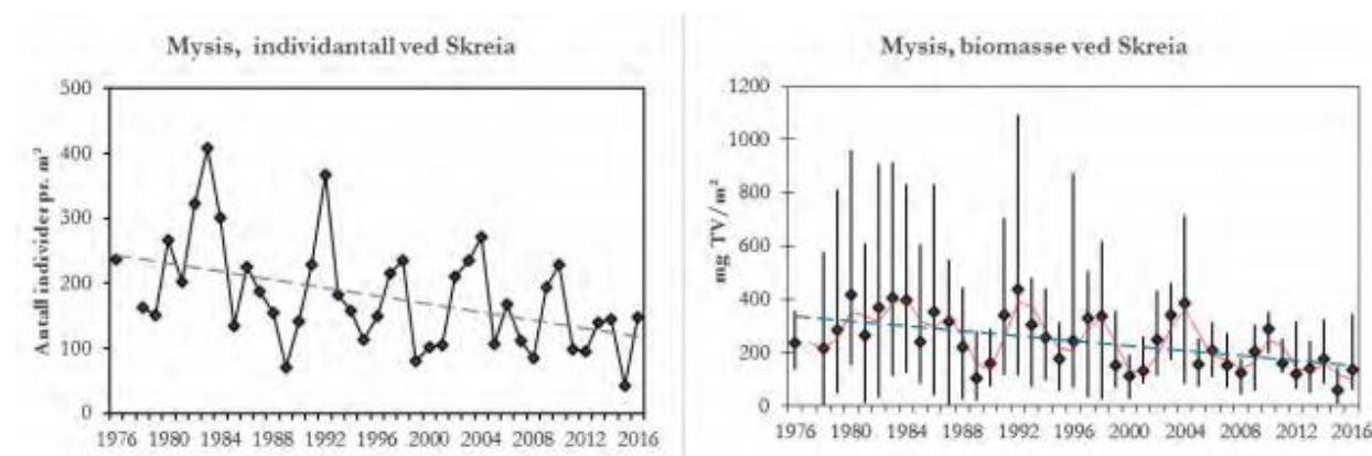
Figur 16. Medelvärden i individtäthet och biomassa av M. relicta vid Skreia (djupaste delen av Mjösa) i perioden 1976-2016. Figurerne är hämtade från Lövik m fl (2017).
