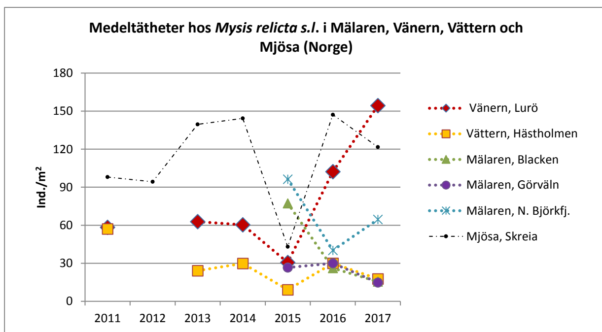
Figur 6. Medeltätheten hos M. relicta s.l. i Mälaren (Blacken, Görvälän, Norra Björkfjärden) 2015-2017 samt i Vänern (Lurö) och Vättern (Hästholmen) 2011, 2013-2017. En jämförelse har också gjorts med tätheter uppmätta vid Skreia i Mjösja (Norge) 2011-2017. Data från Mjösja kommer från övervakningen som NIVA utför på uppdrag från Vassdragsförbundet för Mjösja (Lövik, opubl. se litteraturförteckningen).
