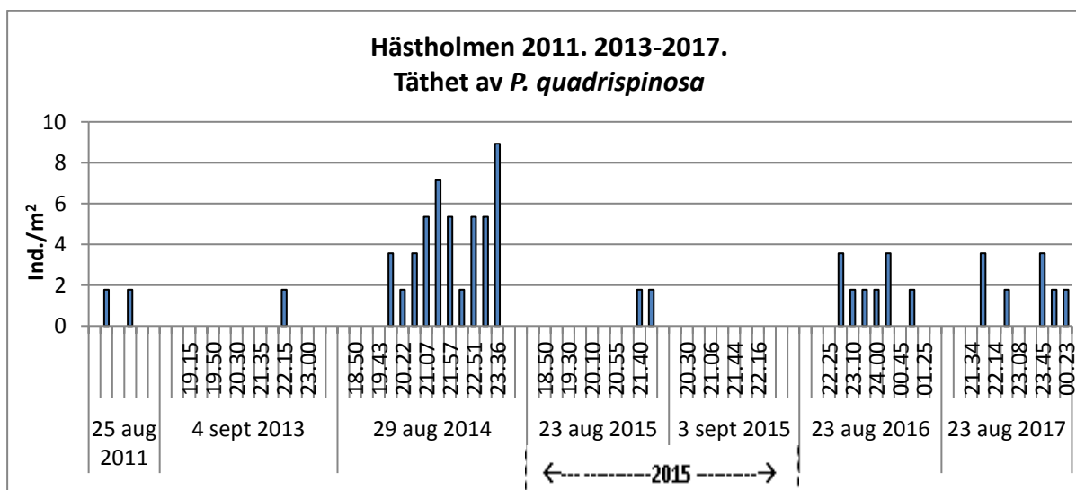
Figur 8. Tätheten av P. quadrispinosa skattad genom håvning över största djupet (100 m) vid Hästholmen, Vättern, vid flera tidpunkter under en kväll i slutet av augusti/början av september 2011, 2013- 2017. (Obs! Två provtillfällen 2015.). Arten påträffades inte vid provtagningen vid Hästholmen den 3/9 2015.
