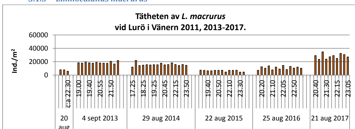
Figur 10. Tätheten av L. macrurus skattad genom hävning vid Lurö, Vänern, över 70 meters djup vid flera tidpunkter under en kväll i slutet av augusti/början av september åren 2011, 2013-2017.
