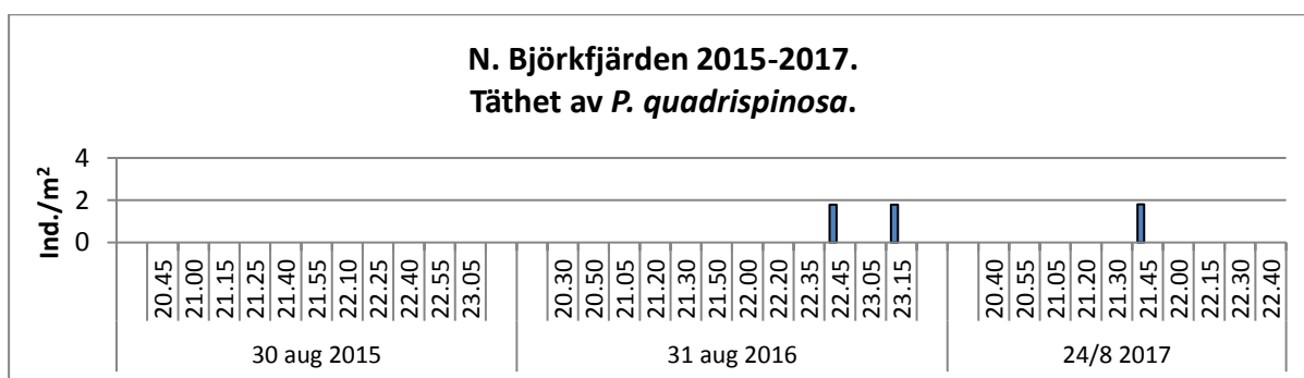
Figur 9. Tätheten av P. quadrispinosa skattad genom håvning i de tre Mälarfjärdarna Blacken, Görväln och Norra Björkfjärden vid flera tidpunkter under en kväll i slutet av augusti/början av september 2015 - 2017.
