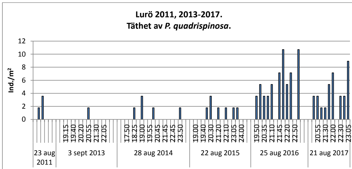
Figur 7. Tätheten av P. quadrispinosa skattad genom håvning över största djupet (70 meter) vid Lurö, Vänern, vid flera tidpunkter under en kväll i slutet av augusti/början av september 2011, 2013- 2017.
