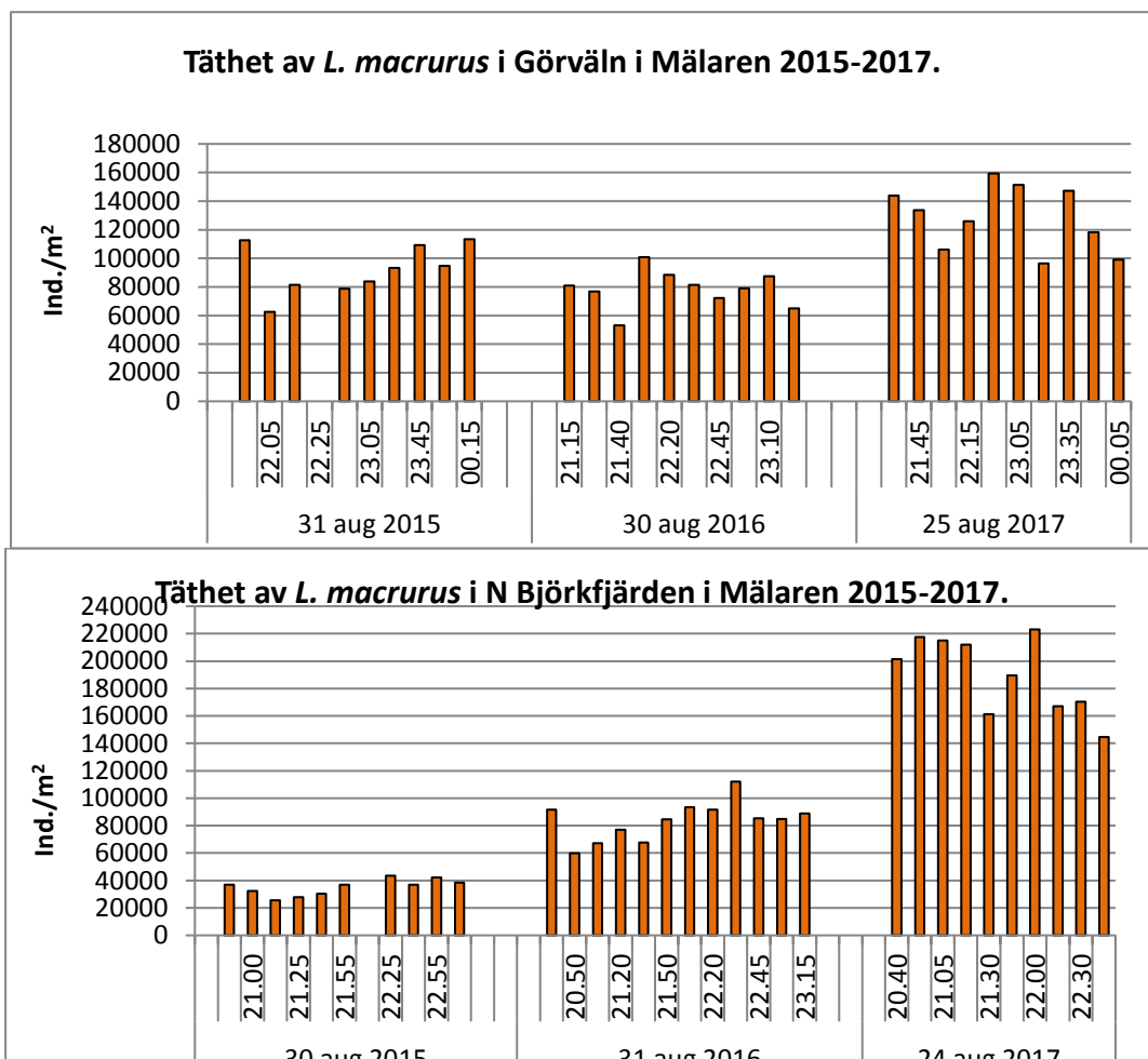
Figur 12. Tätheten av L. macrurus skattad genom hävning i de två Mälarfjärdarna Görväln och Norra Björkfjärden vid flera tidpunkter under en kväll i slutet av augusti 2015 - 2017. Arten har inte påträffats i Blacken 2015-2017.
