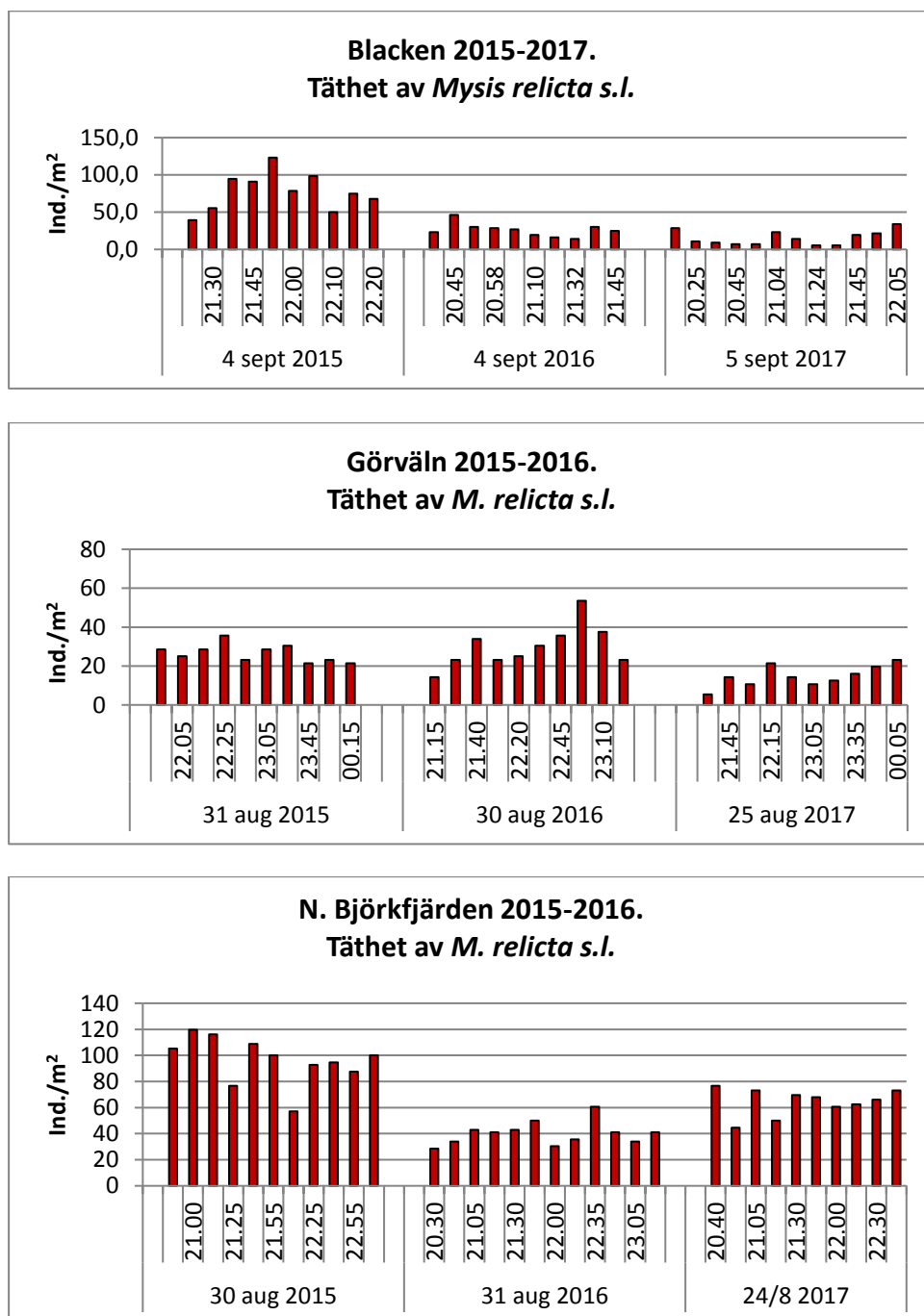
Figur 5. Tätheten av M. relicta s.l. skattad genom hävning över det största djupet i de tre Mälarfjärdarna Blacken (26 m), Görväln (56 m) och Norra Björkfjärden (60 m). Provtagningarna i respektive fjärd skedde vid flera tidpunkter i mörker under en kväll i slutet av augusti/början av september 2015 - 2017.
