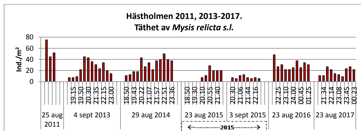
Figur 4. Tätheten av M. relicta s.l. skattad genom håvning över största djupet (100 meter) vid Hästholmen i Vättern. Provtagningarna skedde vid flera tidpunkter under en kväll i slutet av augusti/början av september 2011, 2013-2017. (Obs! Två provtillfällen 2015.)
