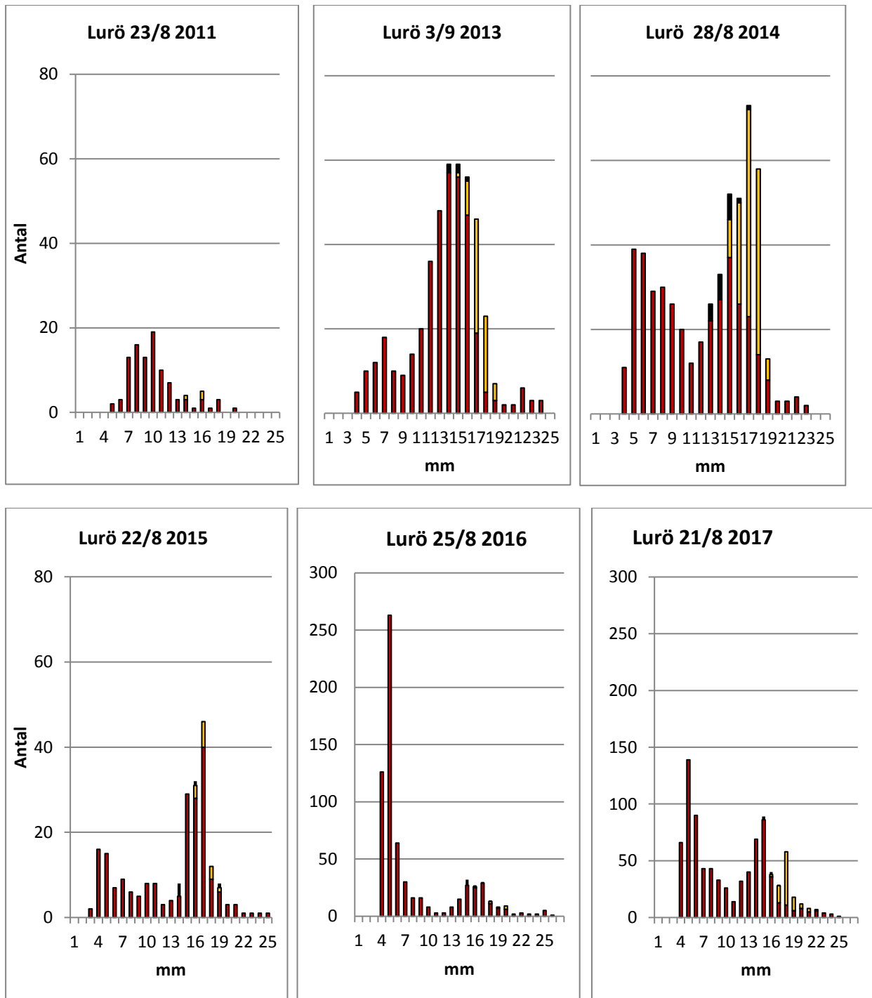
Figur 13. Längdfördelning hos M. relicta s.l. i håvprov insamlade vid Lurö i Vänern över 70 meters djup i slutet av augusti/början av september 2011, 2013, 2014 och 2015. Röd stapel anger juveniler och honor utan embryon, gul stapel anger honor med embryon och svart stapel visar hanar.
