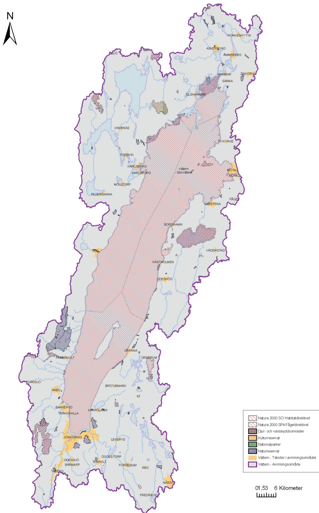
Figur 33. Skyddsområden i Vätterns avrinningsområde.
