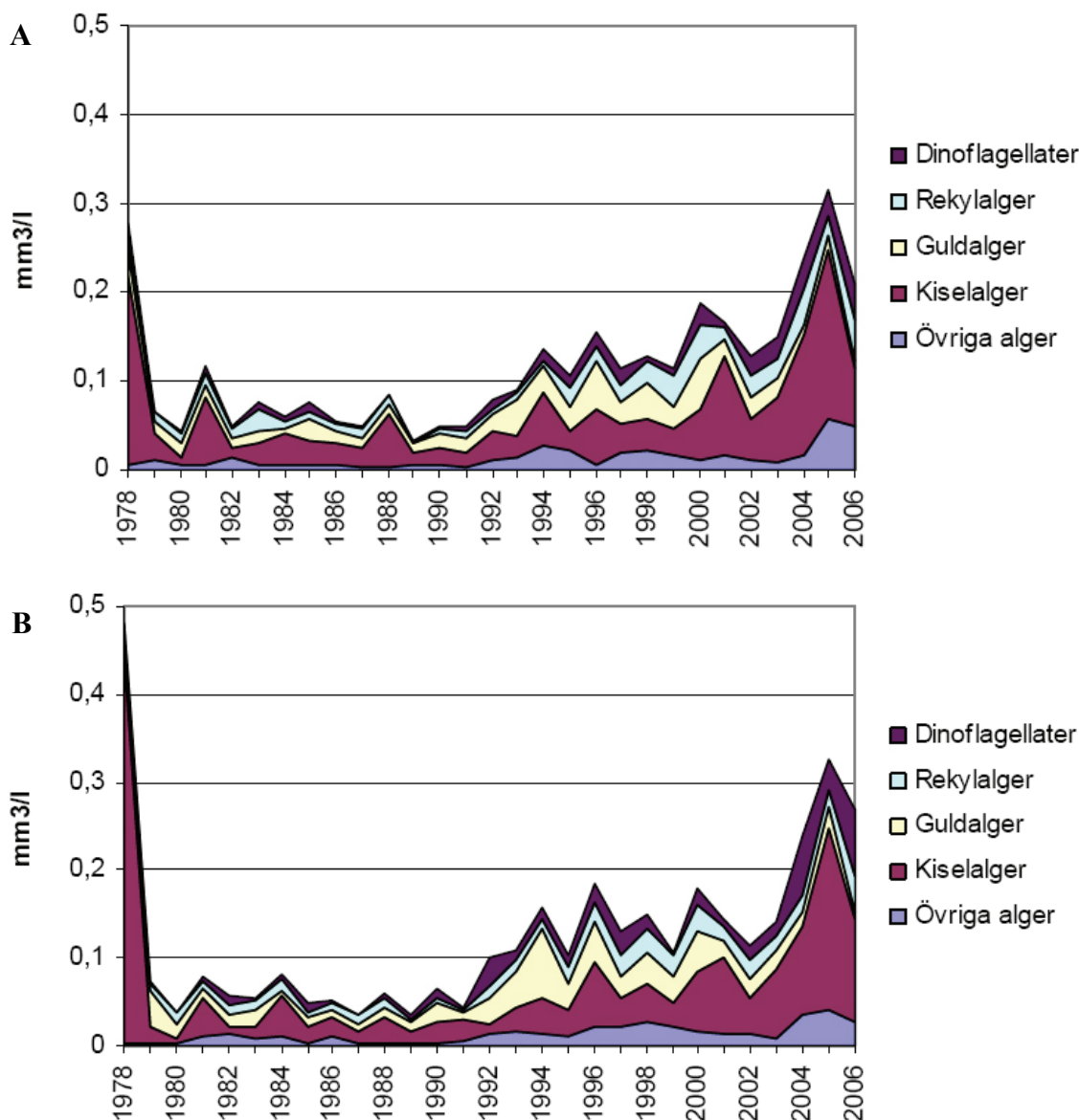
Figur 24. Säsongsmedelvärden av biovolymen ( \text{mm}^3/\text{l} ) för dominerande växtplanktongrupper 1978-2006 vid Edeskvärna (A) i den södra delen av Vättern samt vid Jungfrun (B) i den norra delen av sjön. (Backlund, 2008)
