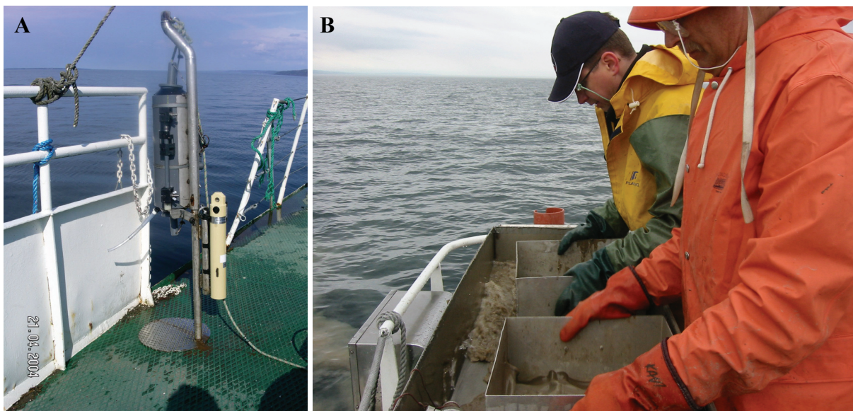
Figur 22. Djupvattenhämtare (A) och sällning av botten sediment (B), (arkivfoto Vätternvårdsförbundet).
