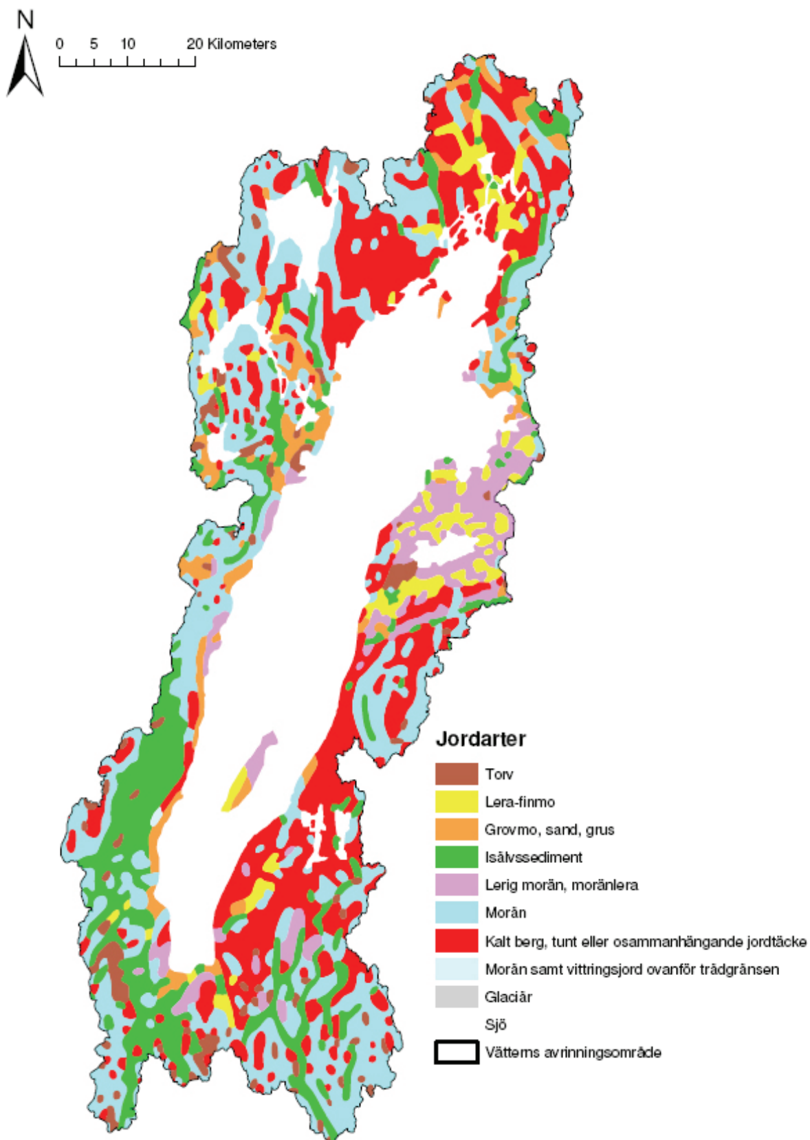
Figur 10. Jordarter i Vätterns tillrinningsområde (Lindell, 2005).
