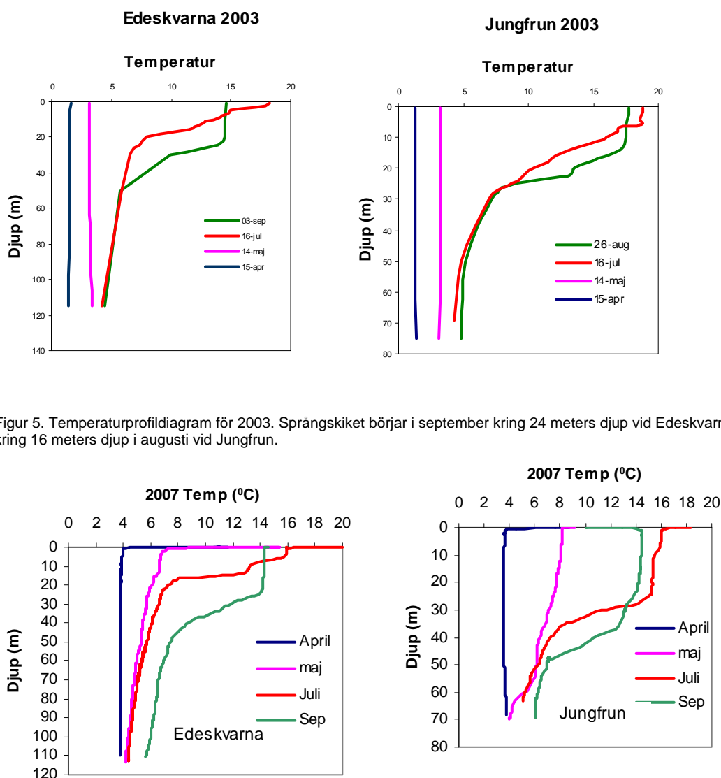
Figur 6. Temperaturprofil diagram för 2007. Språngskiktet börjar i september kring 24 meters djup vid Edesvarna och kring 38 meters djup vid Jungfrun.
